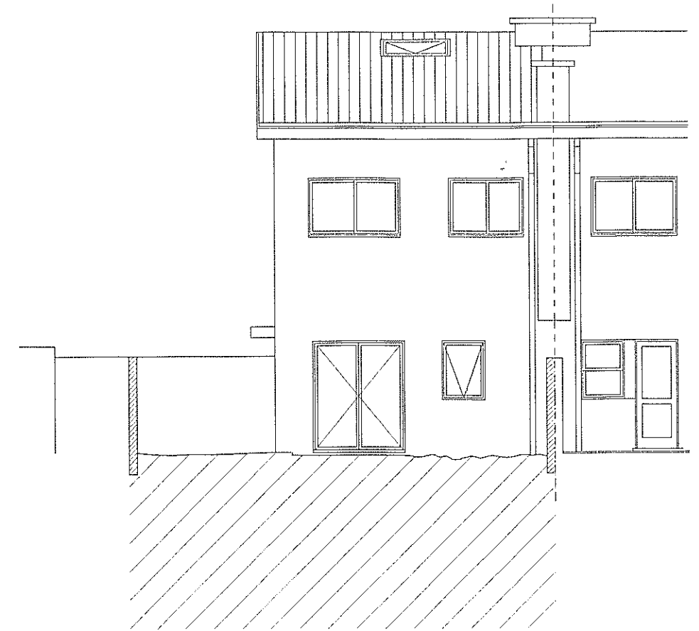
ALÇADO SUL
