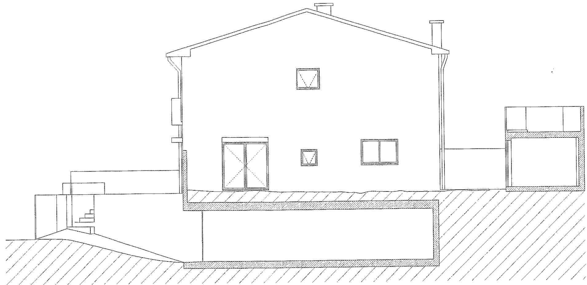
ALÇADO POENTE
